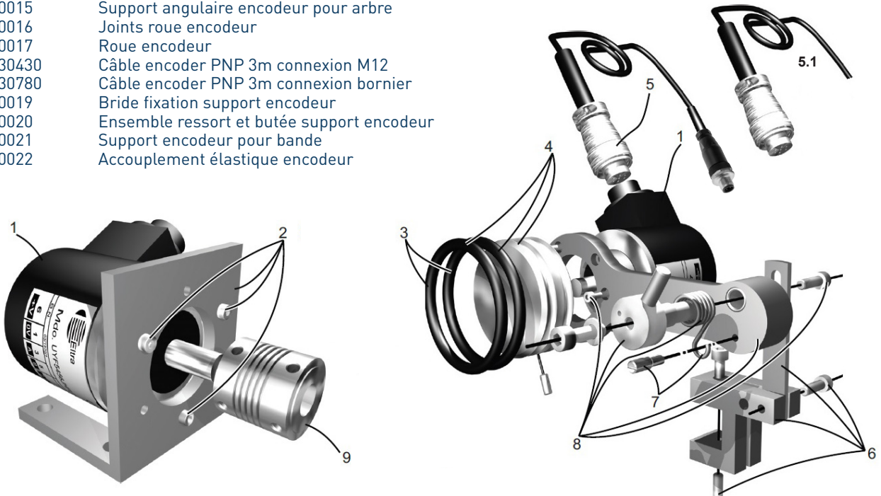
Encodeur pour bande
