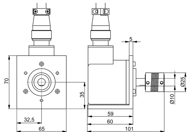
Encodeur pour arbre
